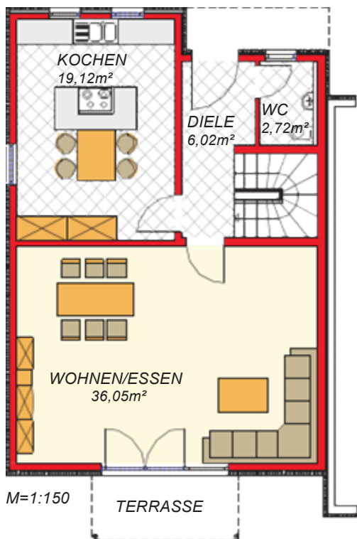
Erdgeschoss VARIANTE C
