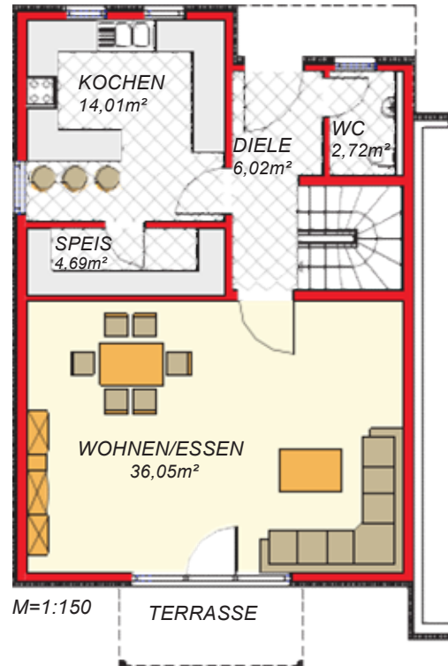
Erdgeschoss VARIANTE B
