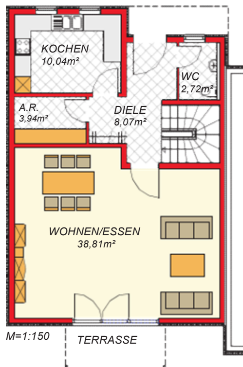
Erdgeschoss VARIANTE D
